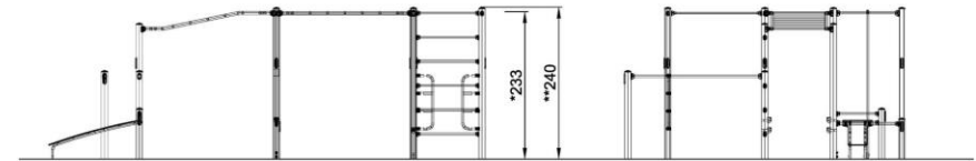
FSW10501 1:100
